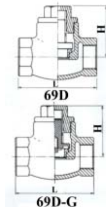
FIG 69D (SUS Disc) FIG 69D-G (Viton Disc)
